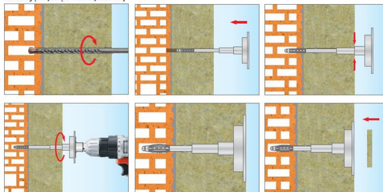
Montaż zagłębiony z krążkiem z wełny mineralnej
